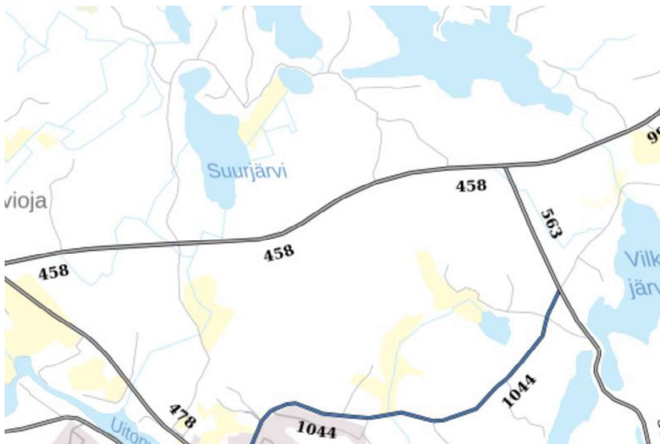
Kuva 9: Ote liikennemääräkartasta
